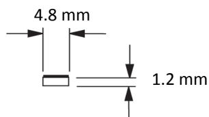
Profilschnitt
